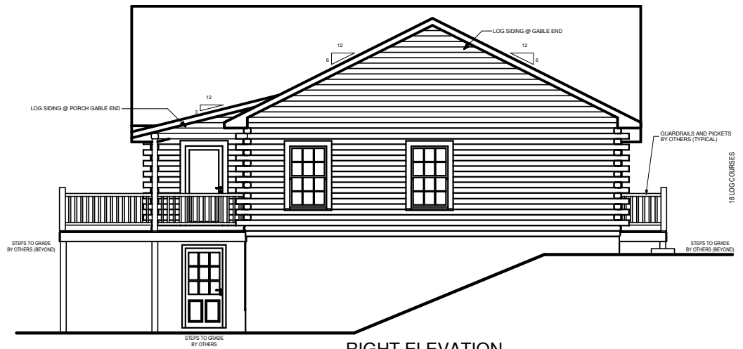
RIGHT ELEVATION
