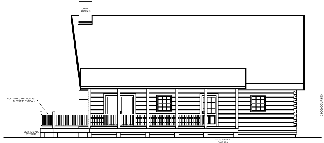
RIGHT ELEVATION
